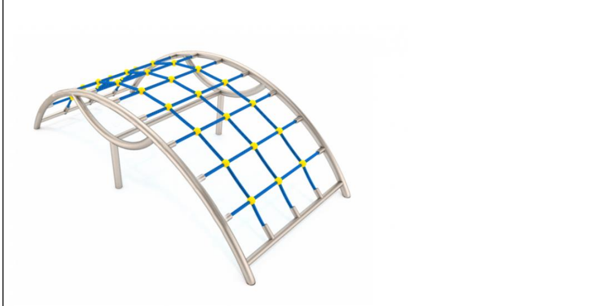
Položka 5 , Šplhací průlezka, materiál kovová konstrukce s lany Bezpečnostní plocha ANO, 20 m 2
